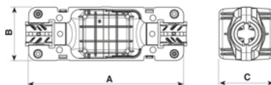
Dimensioni / Dimensions (mm)
